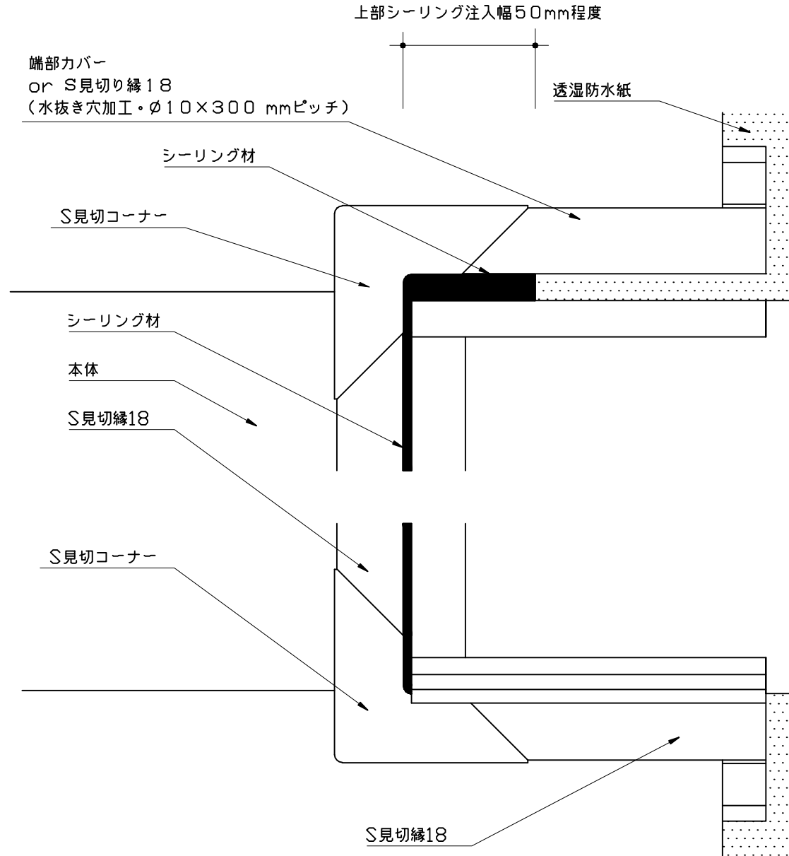
正面納まり図 (左右対称、左側のみ図示)
