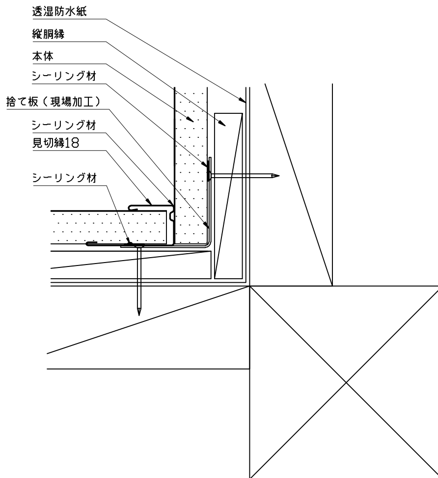
水平断面図
