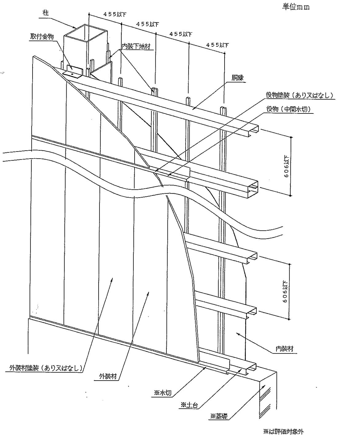
透視図 (胴縁が一般構造用軽量形鋼の場合)
